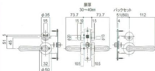
● 製品図 丸座 間仕切錠 LG-G811
