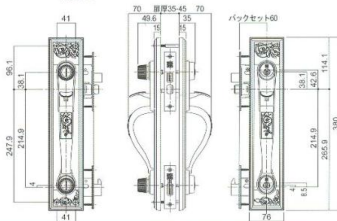
● 製品図 玄関錠ツーロック NF シリンダー KN0156
