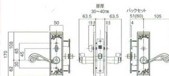
● 製品図 角長座 間仕切錠 LG-G71X
