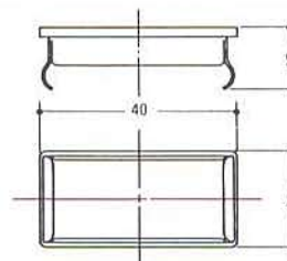
PLUS ST-962 SUS304 Channel Cap
